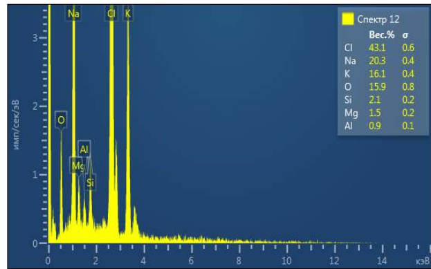
Намуна -5 (-3+1 мм ли фракция)
